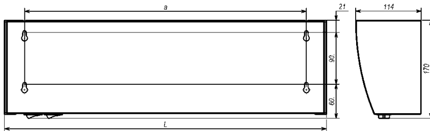
Рис. 2. Габаритные и установочные размеры приборов
